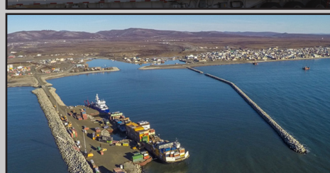
Port of Nome Modification Project
